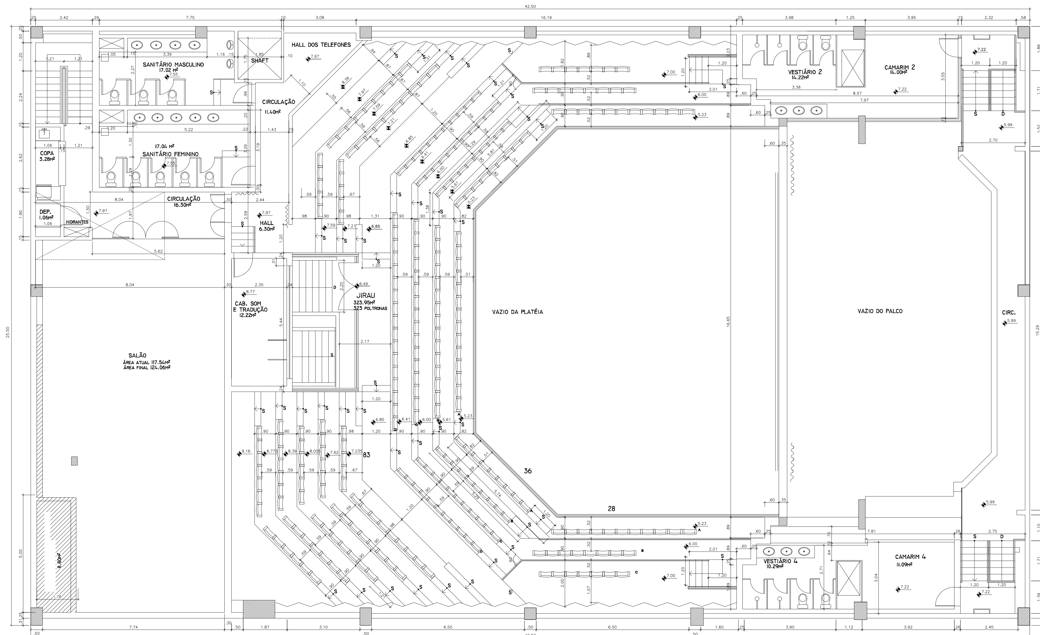
PAVIMENTO SUPERIOR ESCALA 1/75
